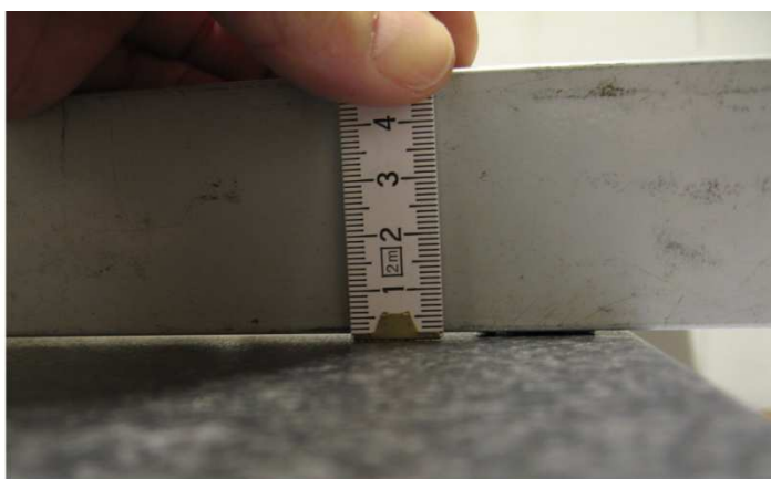
Bordplade måles med tommestok og har en tolerance på 1mm pr. 600mm på tværs, svarende til bordpladens normale dybde og 1mm pr. 1000mm på langs af fronter.
